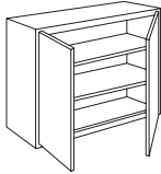
Wall Double Doors Width: 24", 27", 30", 33", 36", 39", 42"
